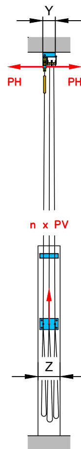
Coupe A-A
