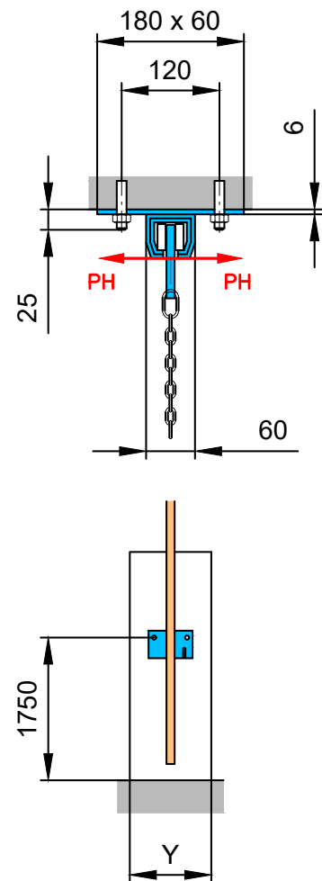
Schnitt A-A
